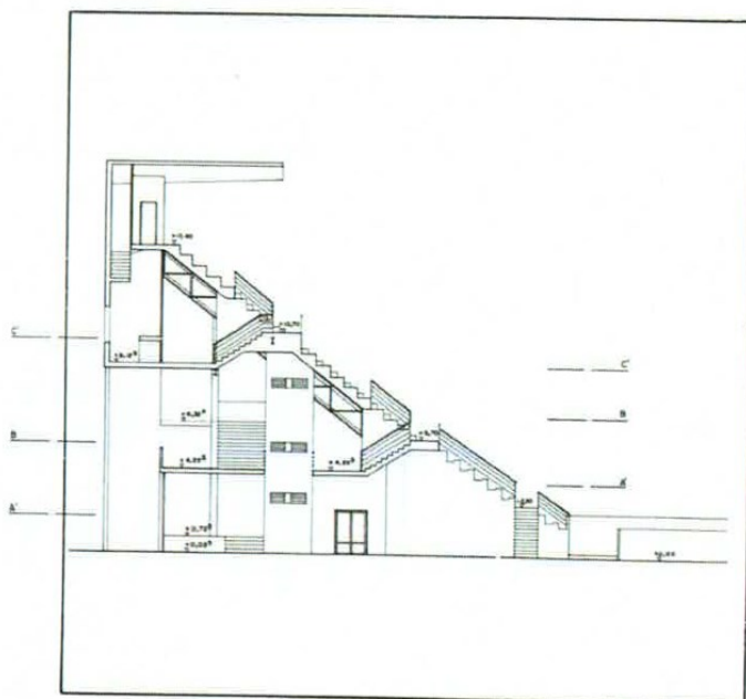
Sección. Acceso presidencia. Proyecto 1989.
